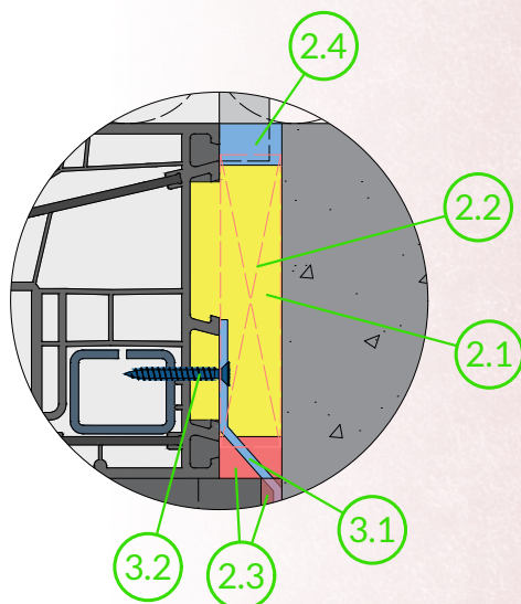
Szczegół B
