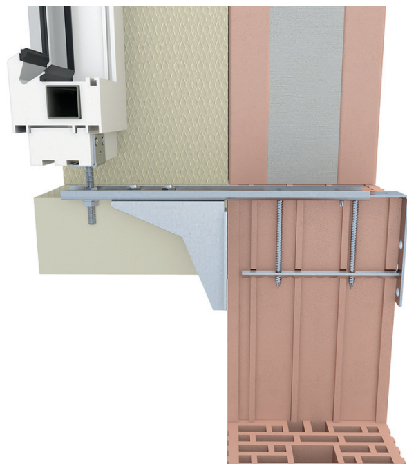
WU-ST-Anker mit Winkelanschluss
